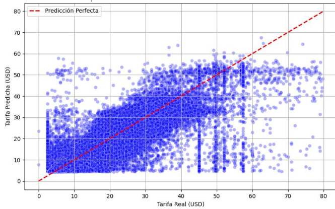
Figura 5: Comparación de valores reales vs predicciones
