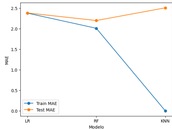
Figura 4: Comparación de error MAE entre entrenamiento y prueba
